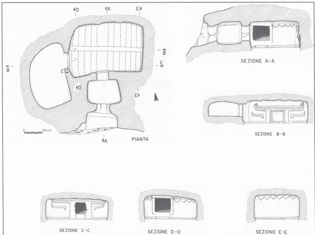
Fig. 1 - La domus istoriata di Sos Baddulesos, (Usini-SS): planimetria e sezioni (dis. di A. Farina). Fig. 1 - The historiated domus of Sos Baddulesos (Usini-SS): plan and sections (drawing by A. Farina).
